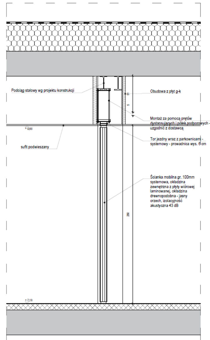
DETAL MOCOWANIA ŚCIANKI MOBILNEJ - 1:20
